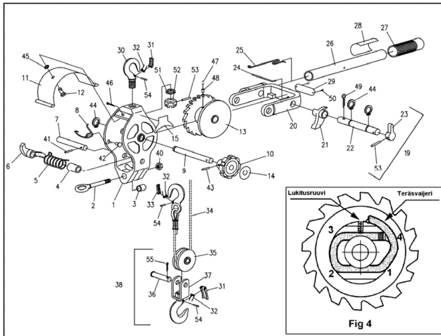
Varaosapiirustus
