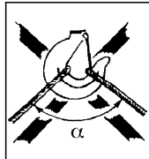
Fig 3 b För stor toppvinkel på slinget! \alpha = \max 60^\circ
