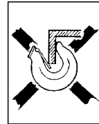
Fig 3 d Krokspetsen dessutom utsatt för böjpåkänning!
