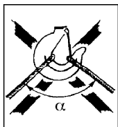
Kuva 3 b Silmukan yläkulma liian suuri! \alpha = enint. 60°
