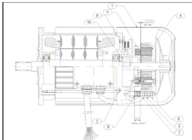
Piirros 11 Jarrullinen kaksinopeusmoottori ABK 101
