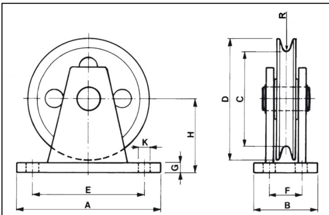
Målskisse – bryteblokk -73
