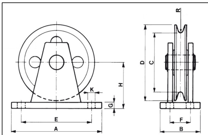
Mittapiirros – väkipyörä -73
