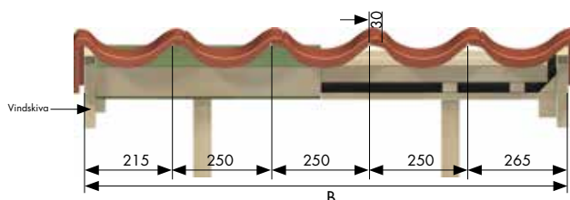
Bild 9b. Gavelpanneindelning för Exklusiv. Separat tabell för mätindelning av tak finns på vår hemsida.
