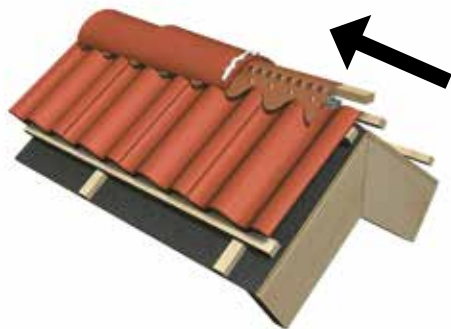
Bild 12. Ventilation av traditionellt papptäckt tak med slutna noken. Benders ventinock är spikad på nockbrädan och tätar mot inblåsande av regn och snö. Samtidigt medges luftcirkulation under takpannorna. Torra tak ruttnar inte! Nockpannorna läggs mot vindriktningen, se pil. Täta och skruva allt spika.
