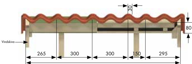
Bild 9a. Gavelpanneindelning för Palema. Separat tabell för mätindelning av tak finns på vår hemsida.
